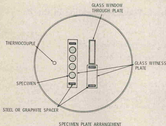
Fig. 1. Specimen-plate arrangement.
